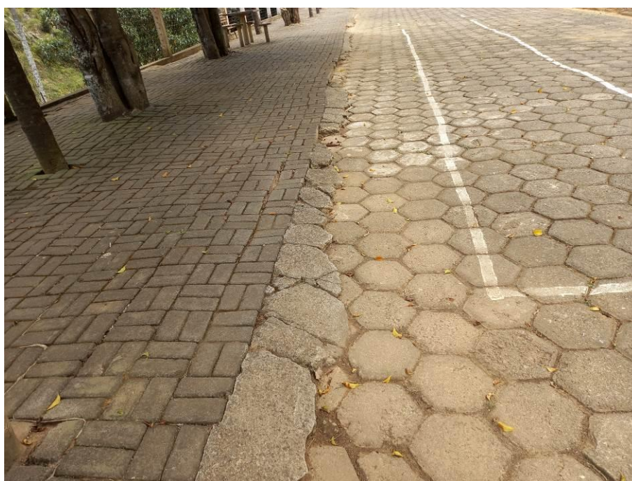
Foto 01: Recomposições com cimento nos pisos intertravados, escurecimento sujidades. Autoria: Alexandra Sales | Data: 16/09/2025
